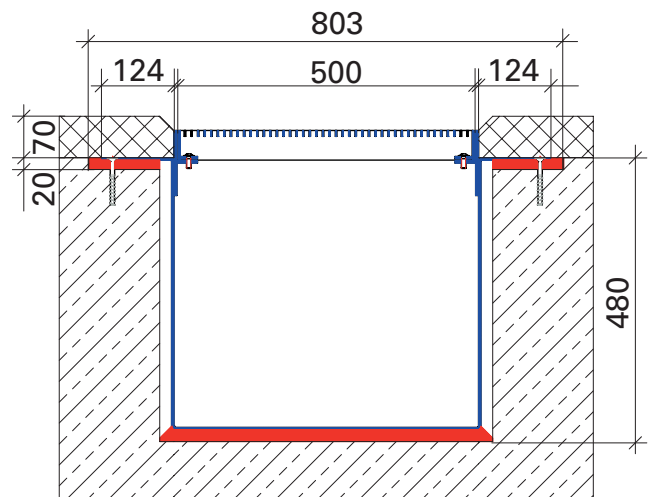
Querschnitt Mulde
