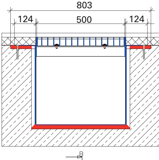
Längsschnitt
